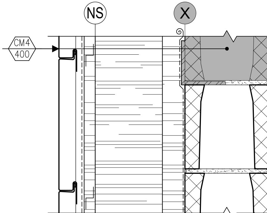
ALLÈGE
