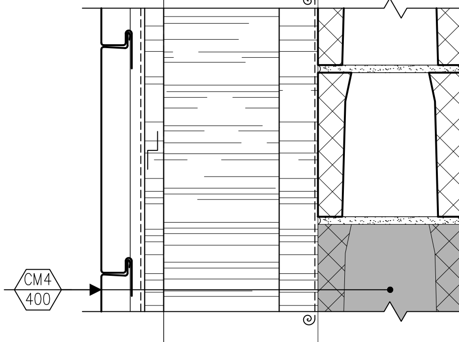
ALLÈGE
