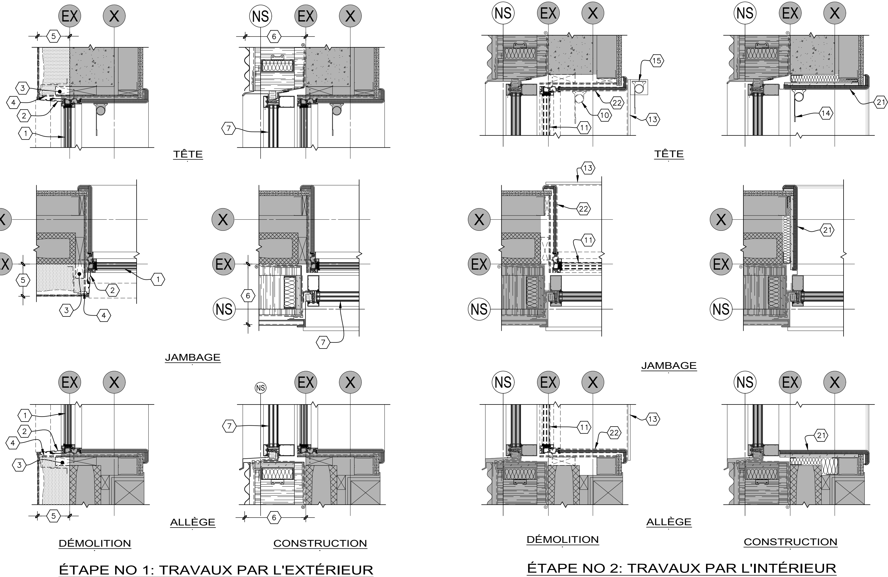
A 502,503 505 PRINCIPE DE REMPLACEMENT DES FENÊTRES DE LA TOUR 1:10mm (NIVEAUX 200, 300 ET 400 - BLOCS DE BÉTON)
