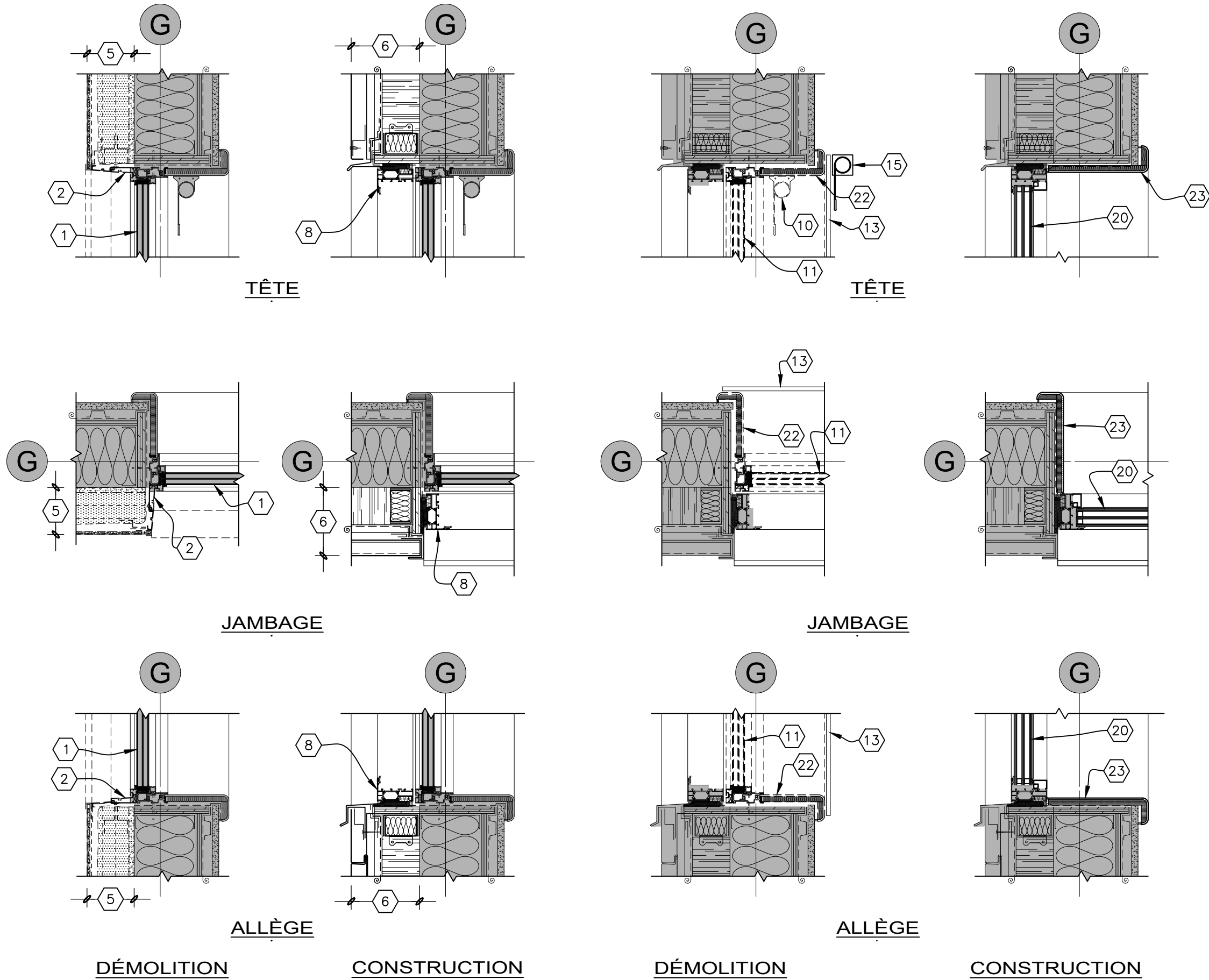
C 502,503 505 PRINCIPE DE REMPLACEMENT DES FENÊTRES DU BASILAIRE 1:10mm (COLOMBAGES MÉTALLIQUES - SECTEUR IRM ET NIVEAU 100)
