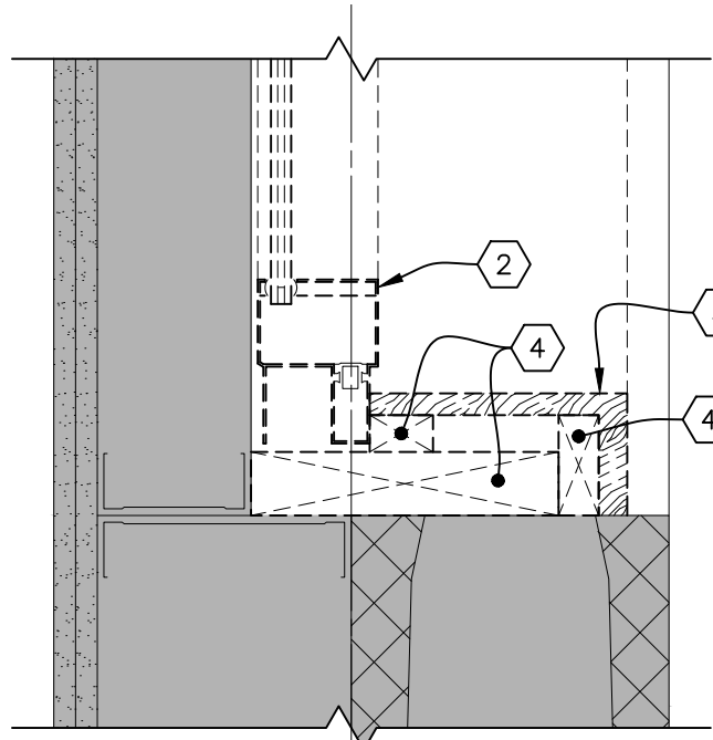
ALLÈGE
