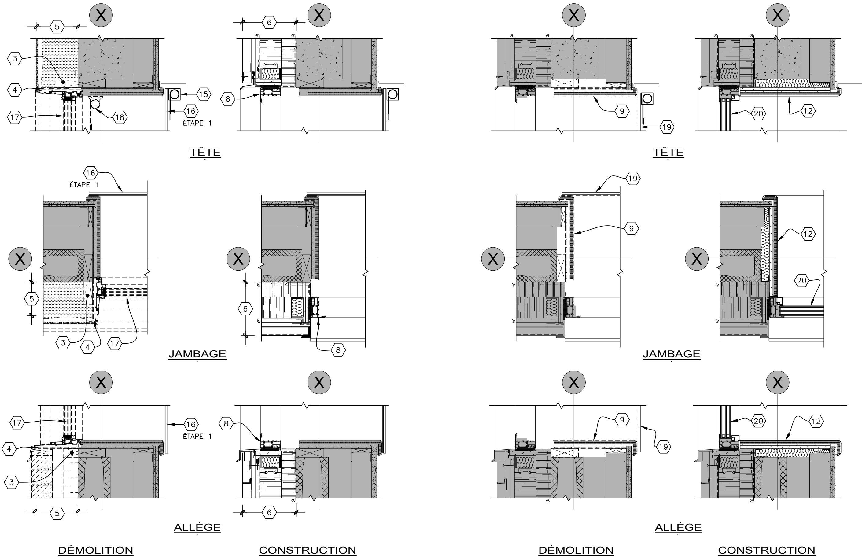
B 502,503 505 PRINCIPE DE REMPLACEMENT DES FENÊTRES DU BASILAIRE 1:10mm (NIVEAU RDC - BLOCS DE BÉTON - EXCLUANT SECTEUR IRM)
