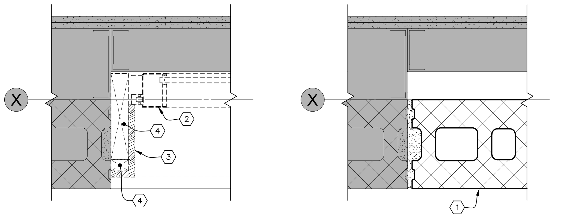
JAMBAGE
