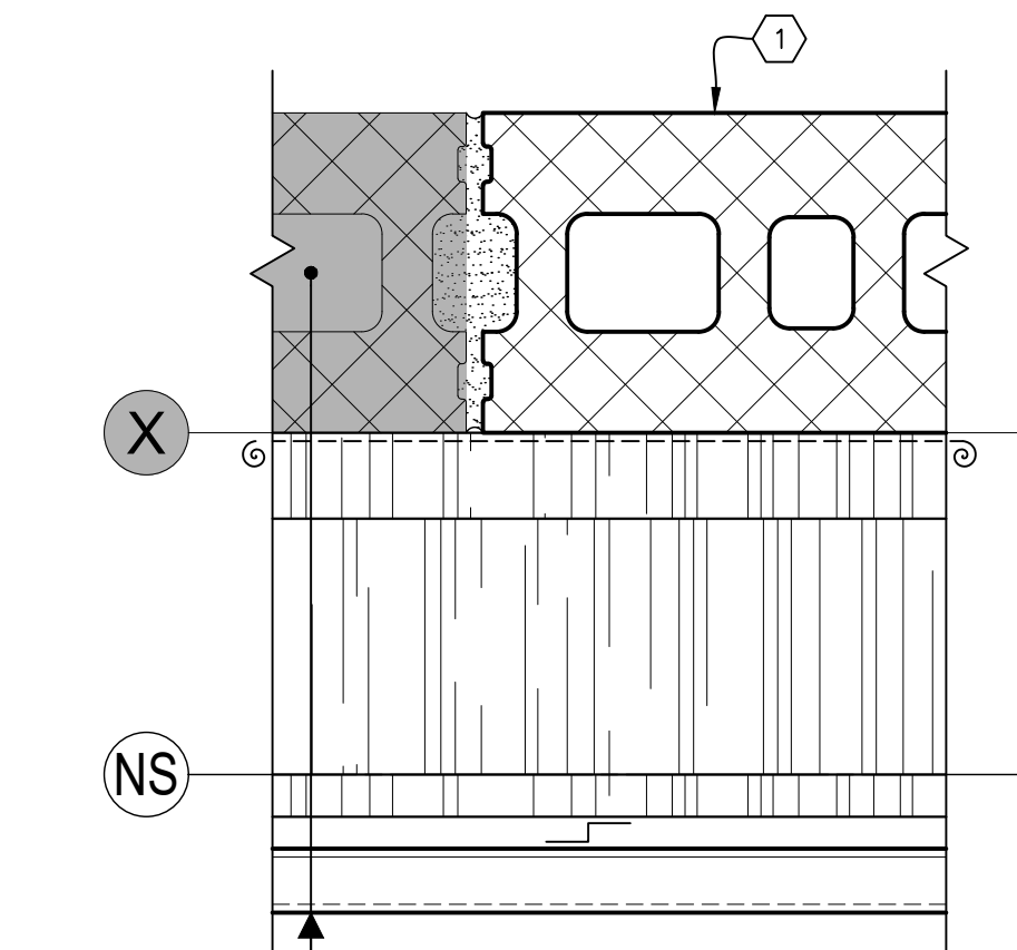
TÊTE
